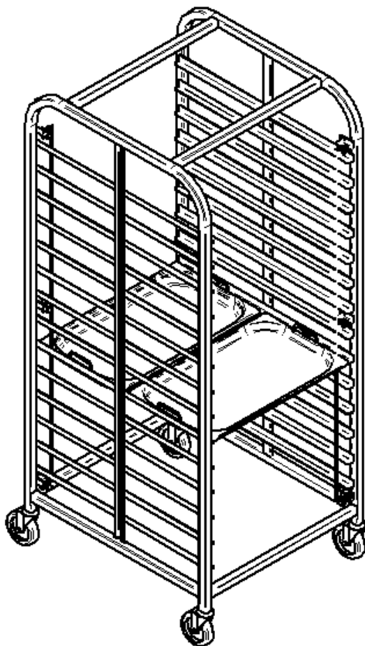
Рис.5 ТШГ-14-2/1
