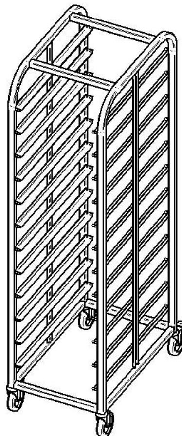
Рис.6 ТШГ-12
